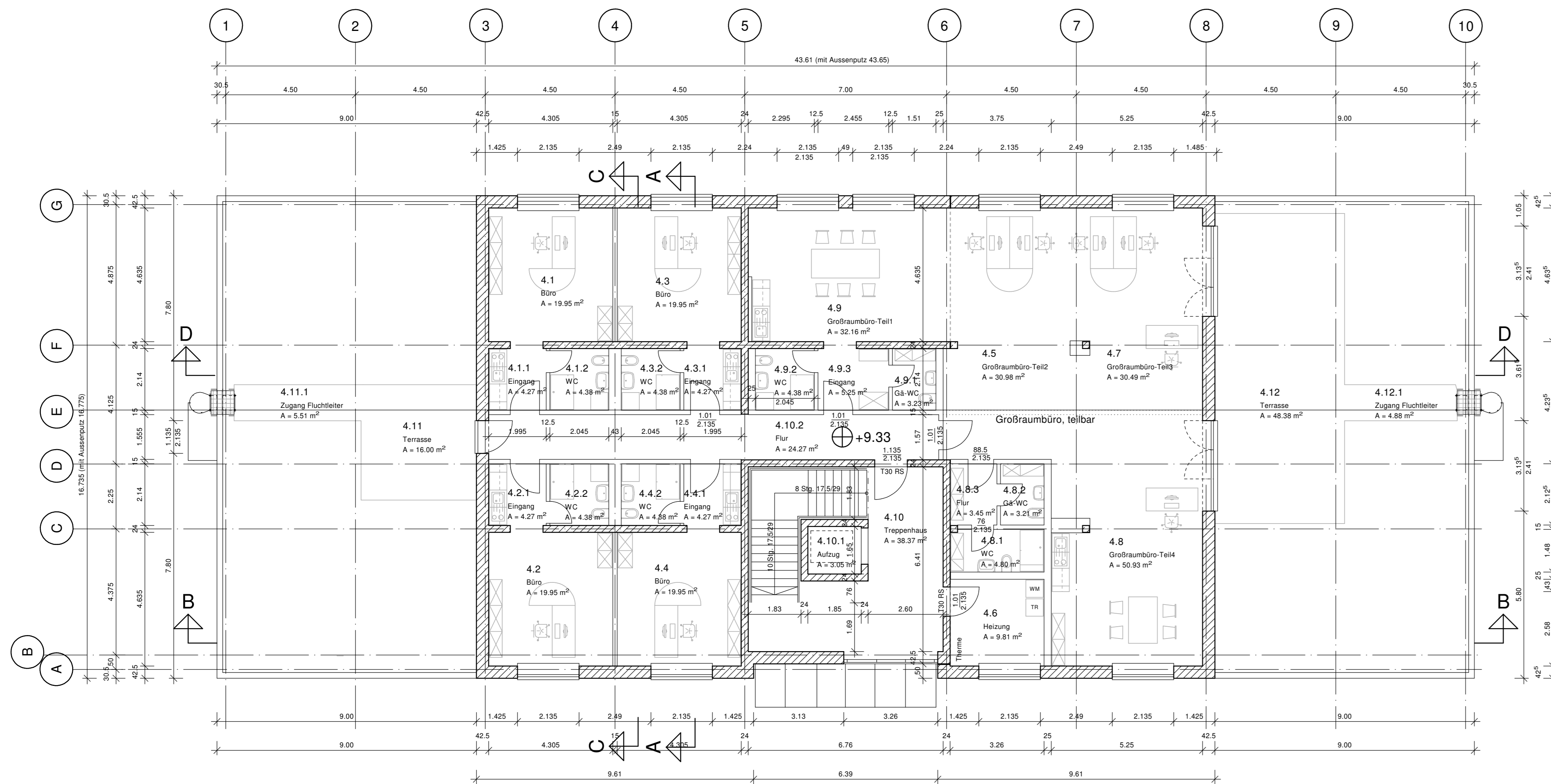
3. Obergeschoss insg. 5 Büros (davon 1 Großraumbüro/ teilbar), 424.71 m² BGF, 358.78 m² NGF, 224.36 m² Bürofläche, 74.77 m² Terrasse mit Zugang Fluchtleiter
