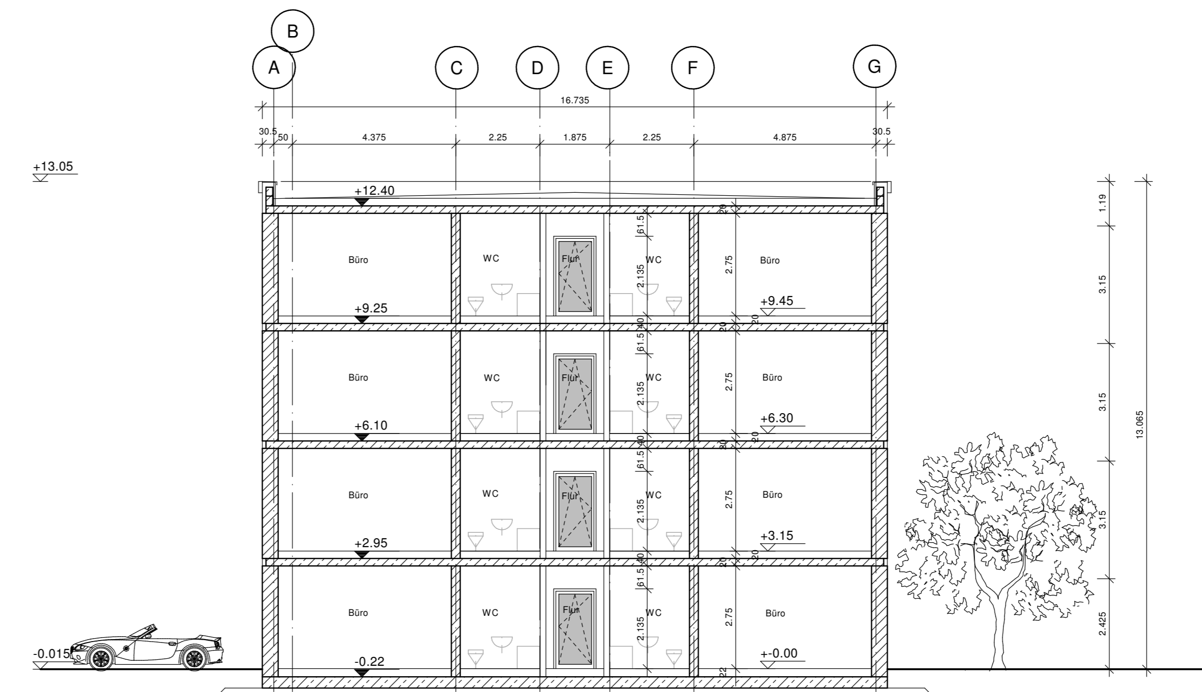
Schnitt C-C
