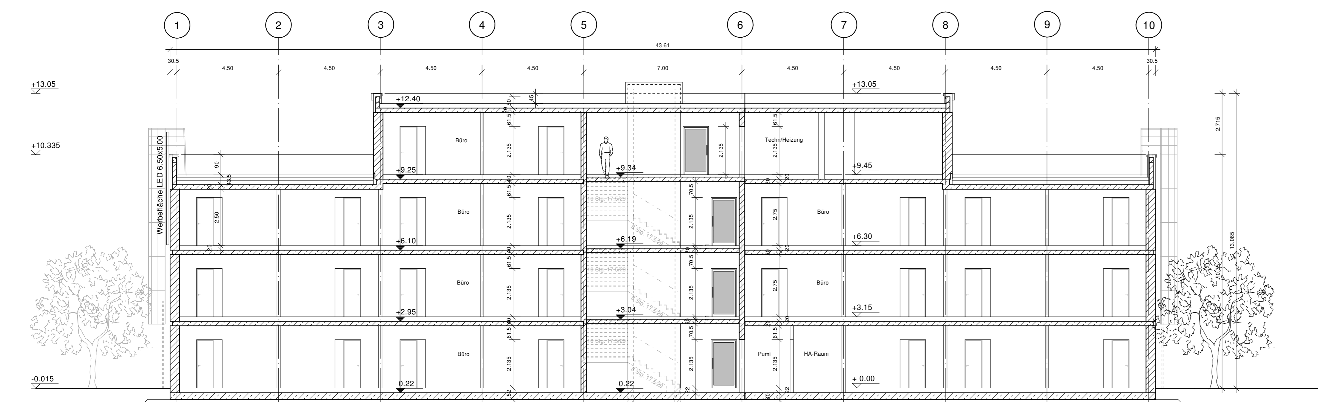
Schnitt B-B
