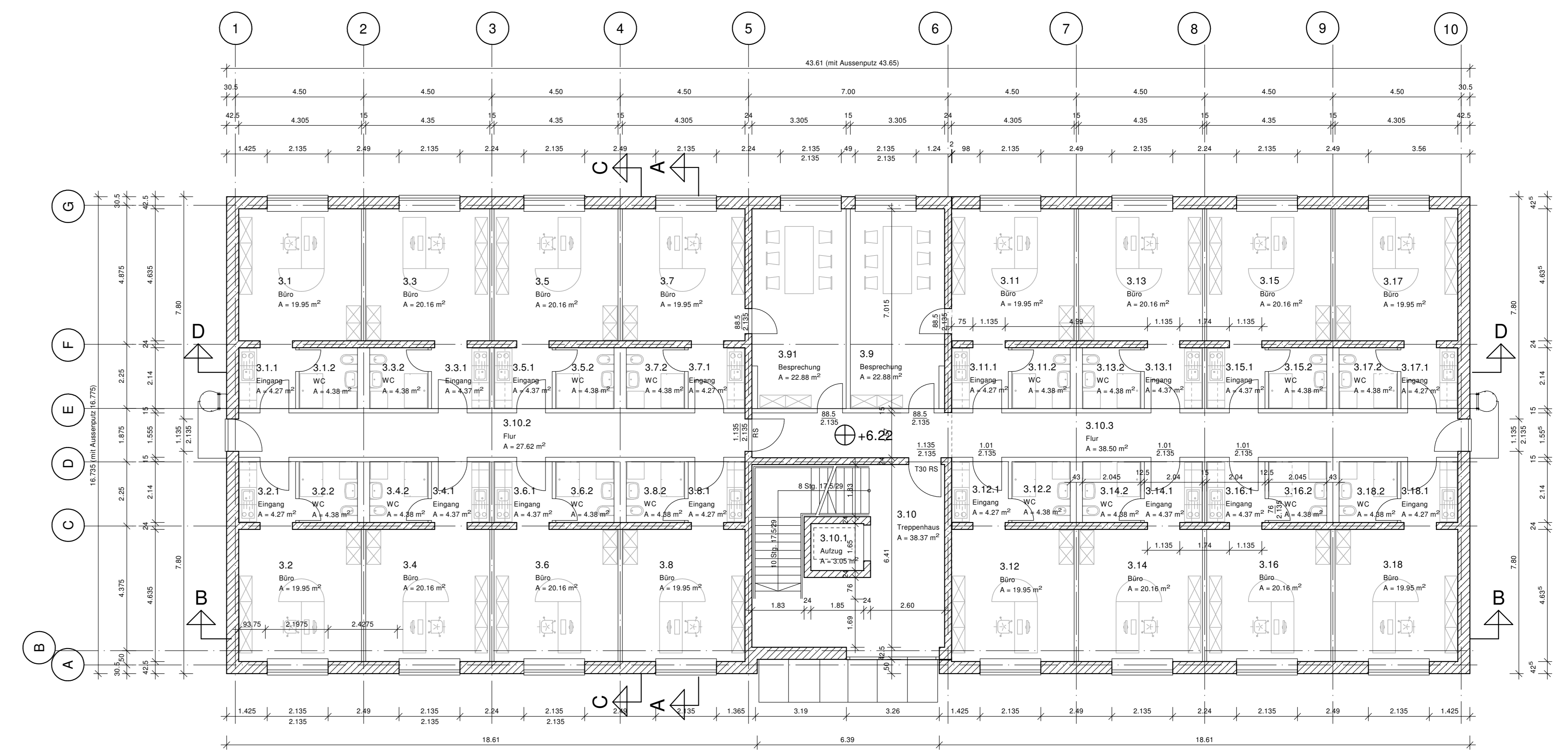
2. Obergeschoss insg. 16 Büros (davon 2 2-Zimmerbüro), 728.51 m² BGF, 613.38 m² NGF, 366.64 m² Bürofläche
