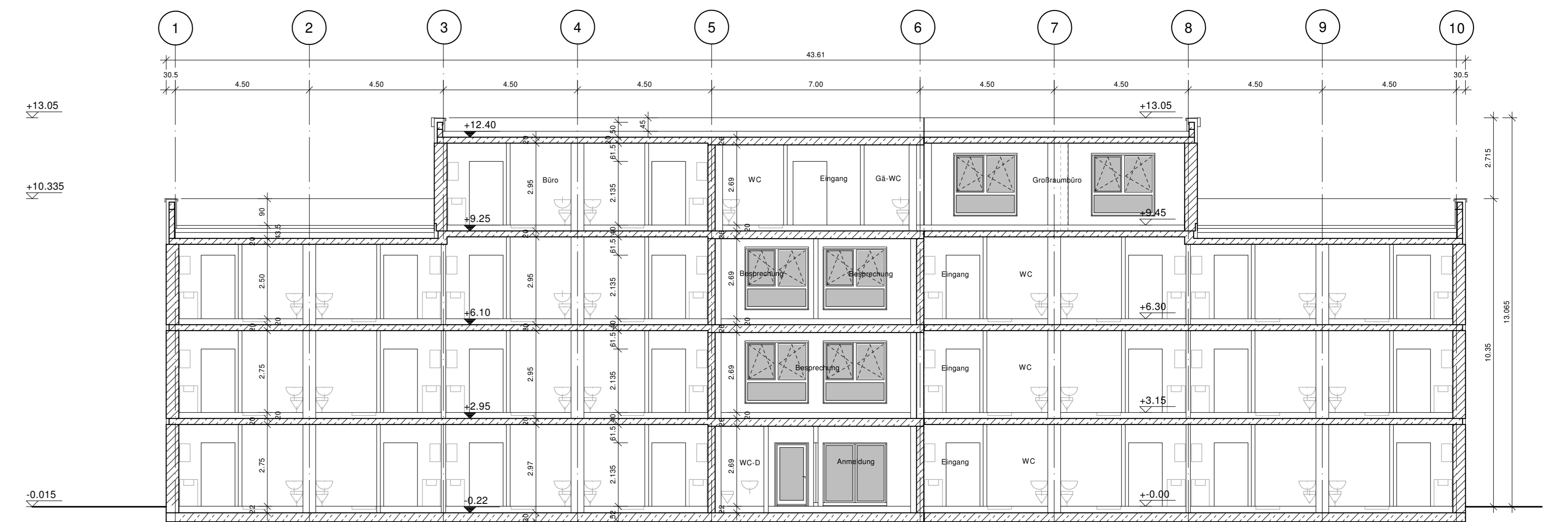
Schnitt D-D
