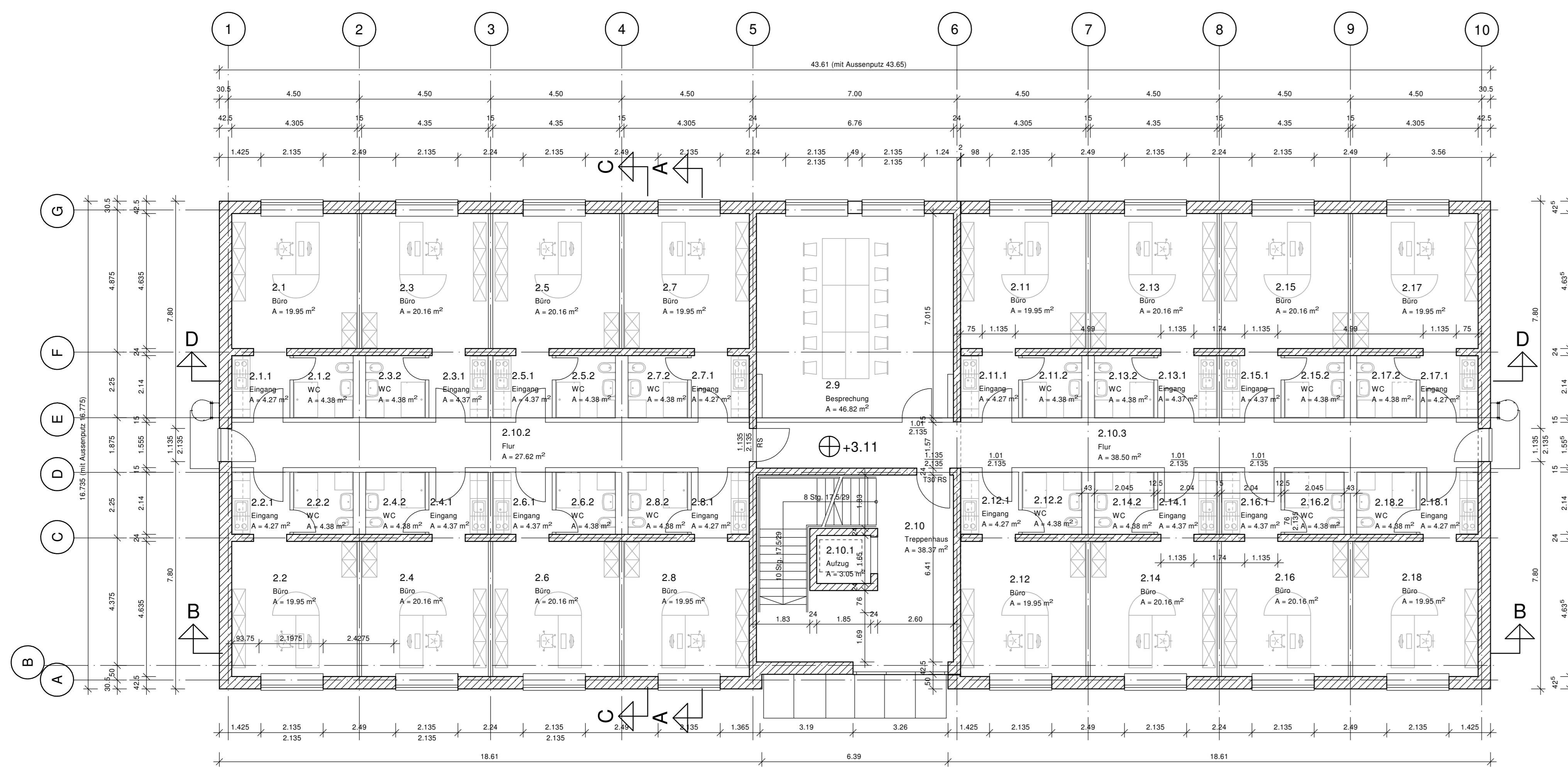
1. Obergeschoss insg. 16 Büros, 728.51 m² BGF, 614.44 m² NGF, 367.70 m² Bürofläche
